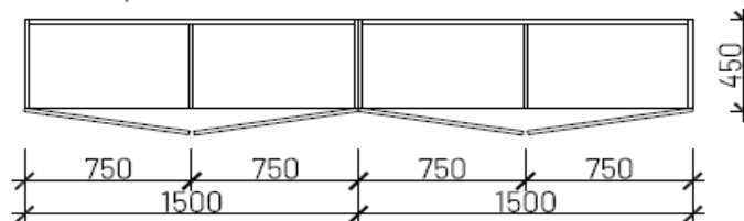
vodorovný řez 2
