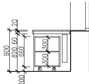
řez b
