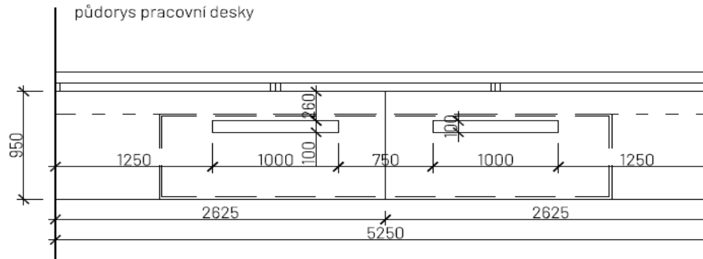
půdorys pracovní desky
