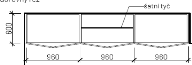
vodorovný řez
