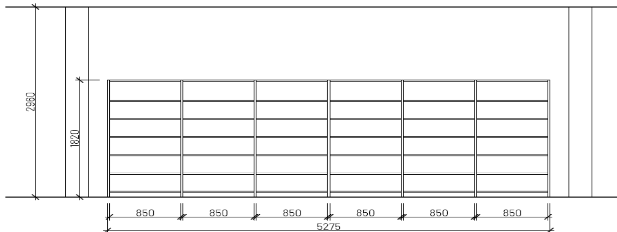
pohled
