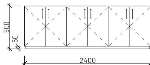
půdorys
