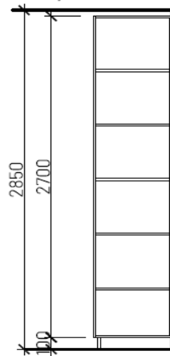
svislý řez
