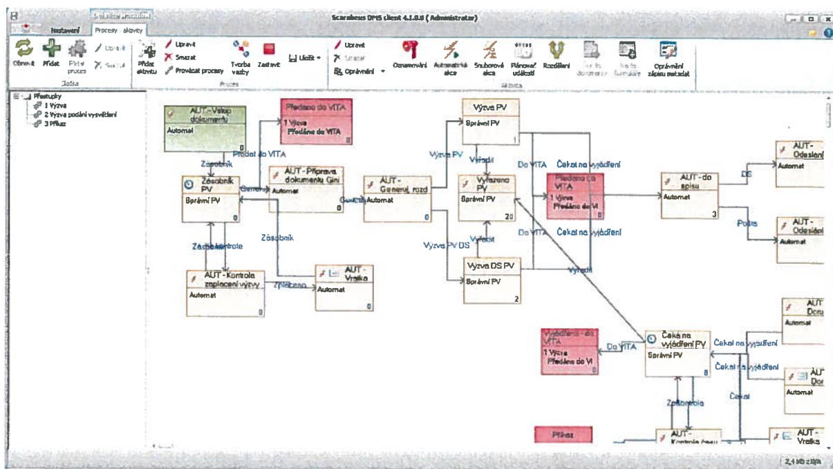
Obrázek 2 Definice procesu zpracování přestupků
